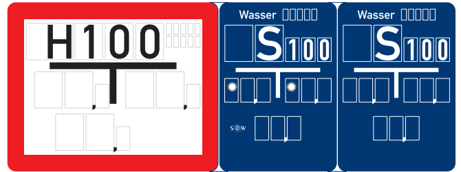
Hinweisschild Kombination Hydrant u. Schieber 2-fach mit 10 bzw. 5 Nummerierungsfeldern
