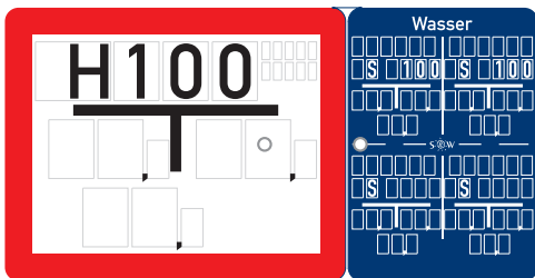
Hinweisschild Kombination Hydrant u. Schieber 4-fach mit 10 Nummerierungsfeldern
