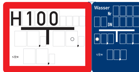
Hinweisschild Kombination Hydrant AX u. Schieber AX mit 5 Nummerierungsfeldern
