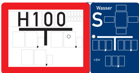
Hinweisschild Kombination Hydrant u. Schiebergruppe mit 10 Nummerierungsfeldern
