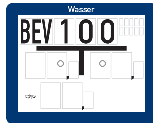
Be- und Entlüftungsventil Aufdruck „BEV100; Wasser“ mit 10 Nummerierungsfeldern
