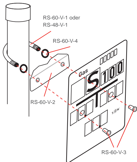
Montageanleitung Rundbügelschelle RS 60 V und RS 48 V
