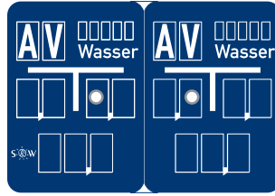
Hausanschluss Wasser 2-fach n. DIN 4067 C mit 5 Nummerierungsfeldern
