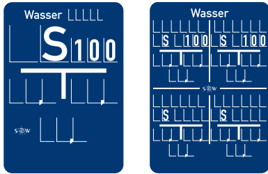
Folienschild Wasser-Schieber 1-fach n. DIN 4067 B
