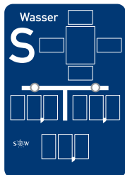
Hinweisschild für Schiebergruppe mit Feld für Lageangaben (als Symbole) und Dimensionsangaben
